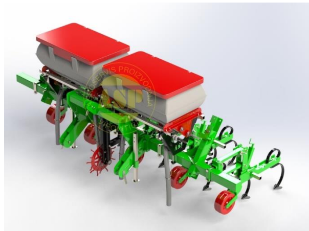
Međuredni kultivator STRCC 4
